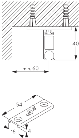
SG 6124 Steun
