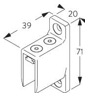
SG 6614 Wandsteun, metaal
