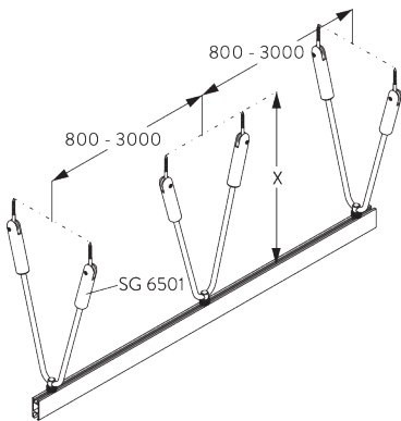
SG 6501: V pendel zorgt voor extra laterale stabiliteit.
