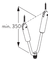
SG 6501 V-pendel
