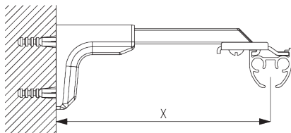
Universal Smart Fix SG 11154 - SG 11156 en steun SG 3832: Schroef SG 10407 (M4x10) nodig.
